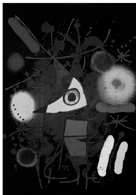
(d) Saturation
